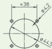
Gatmaat SCHUKO
