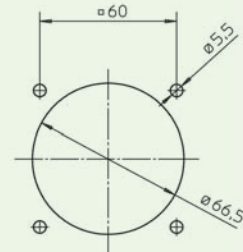
Gatmaat CEE
